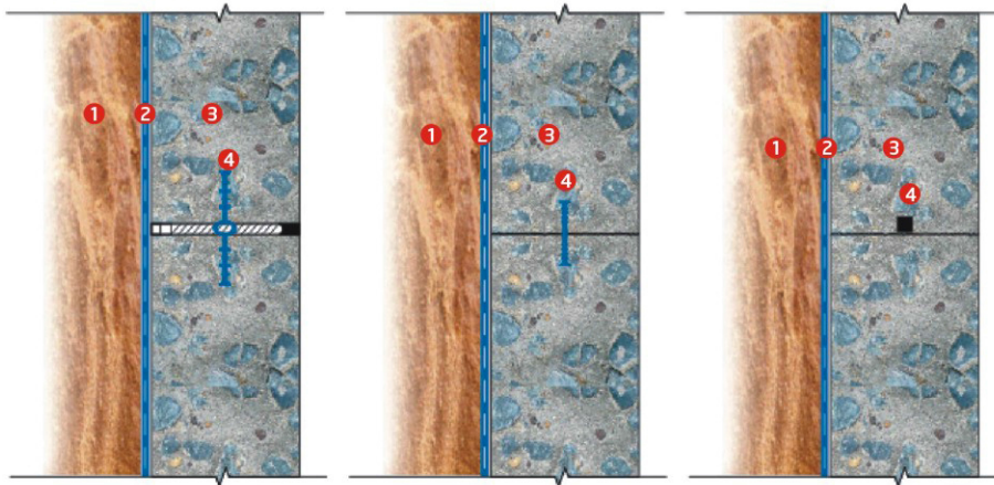
WALL JOINT & RETAINING WALL Khe & Tường chắn đất
