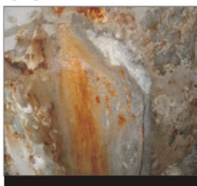
Leakage at construction joint Thấm nặng trên tường chắn đất & mạch ngừng
