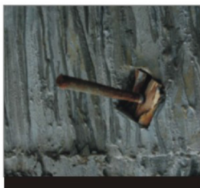
Coin holes, tie bar & protruded steel on the wall Lỗ ty, sắt chò, sắt lồi trên tường chắn đất tầng hầm
